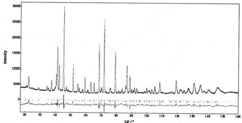
図 2. 測定した中性子粉末回折データ
