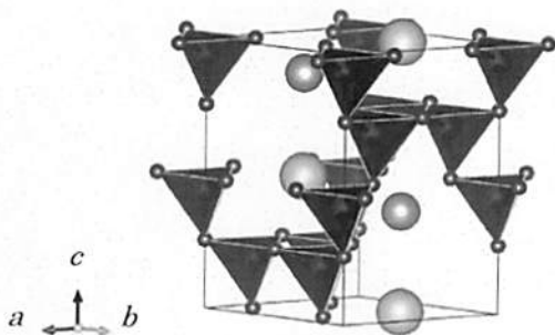
図 1. カゴメ構造を有する YBaCo 4 O 7 系材料の結晶構造
